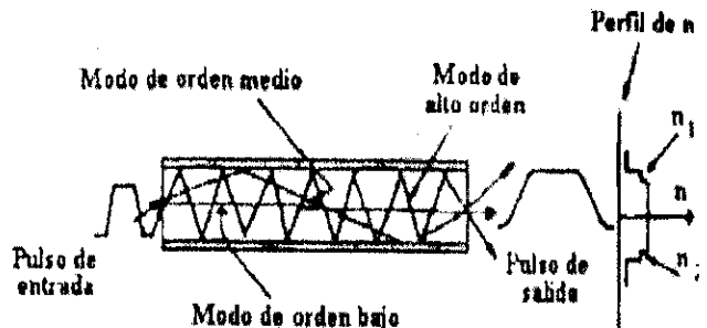
Figura 1. Fibra Multimodo de índice Abrupto
