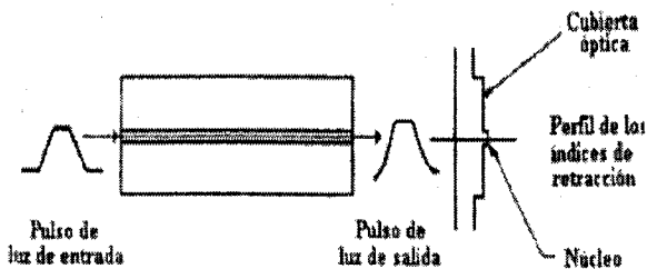
Figura 3. Dispersión Cromática y Perfil del Índice de Refracción
