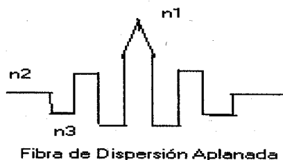
Figura 5. Perfil de una Fibra de Dispersión Aplanada
