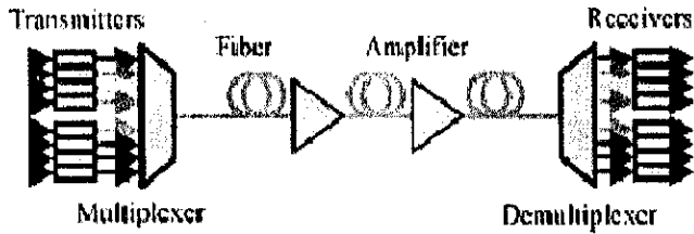
Figura 12. Sistema DWDM
