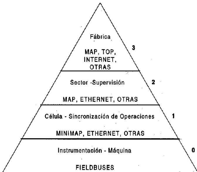
Figura 2 – CIM y protocolos de redes que agrupa
