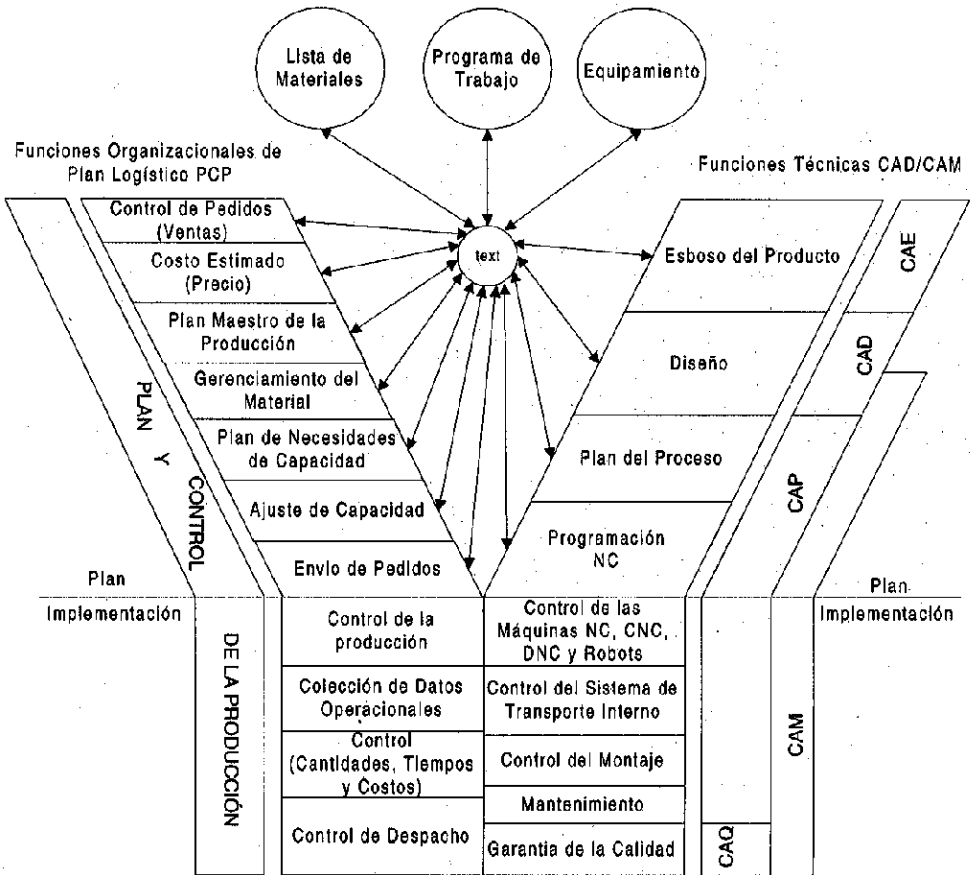
Figura 1 – Modelo Y del sistema CIM
