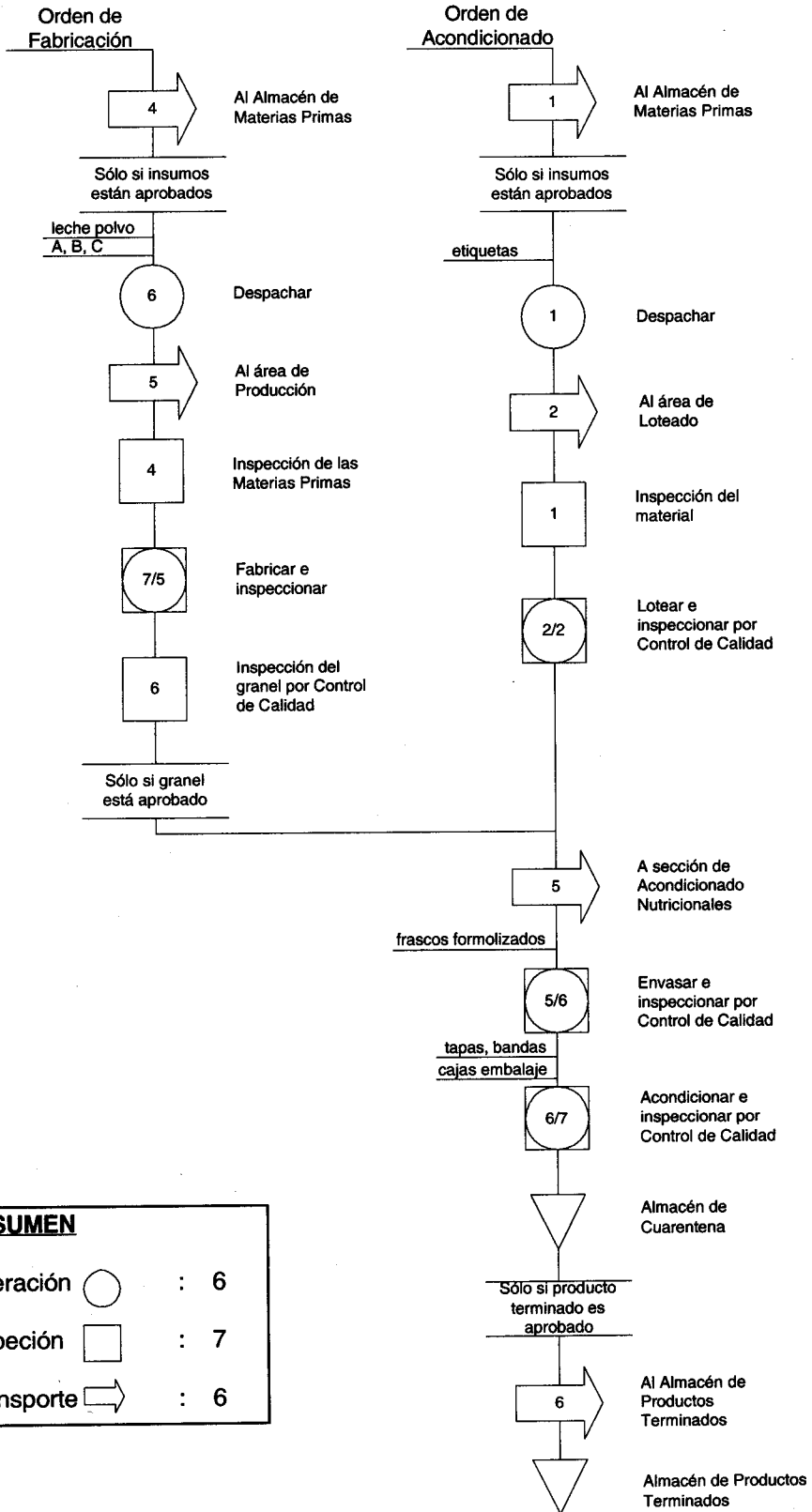
GRAFICO 2.6. PROCESO DE FABRICACION DE NUTRICIONALES
