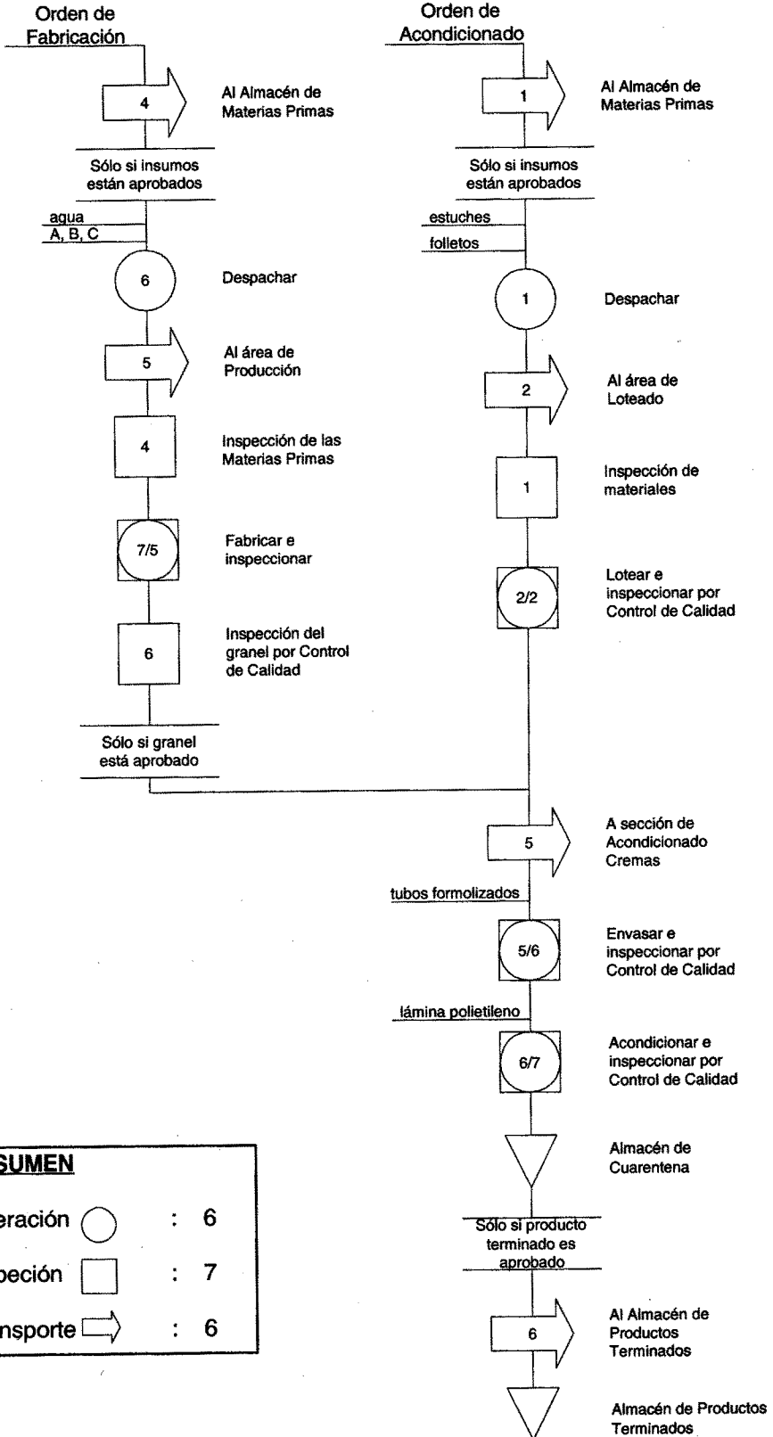
GRAFICO 2.5. PROCESO DE FABRICACION DE CREMAS
