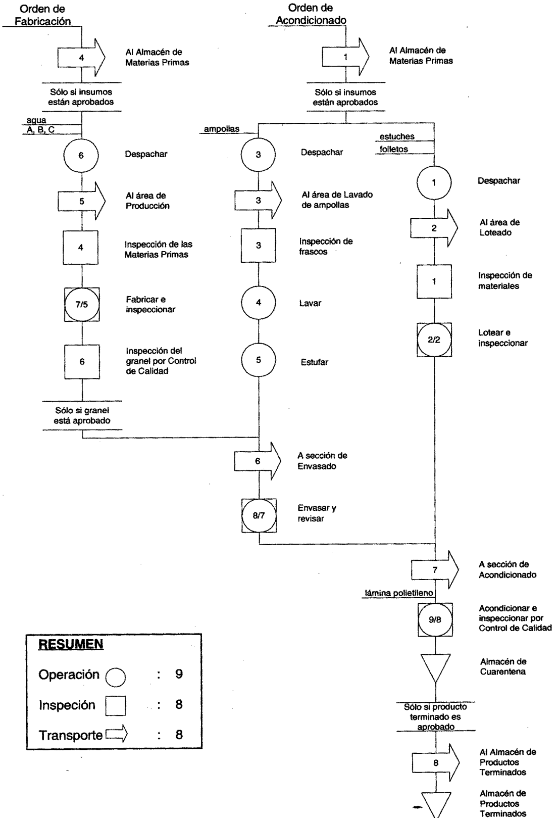
GRAFICO 2.4. PROCESO DE FABRICACION DE INYECTABLES
