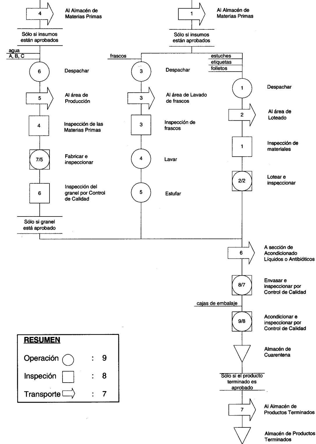
GRAFICO 2.3. PROCESO DE FABRICACION DE JARABES-SUSPENSION
