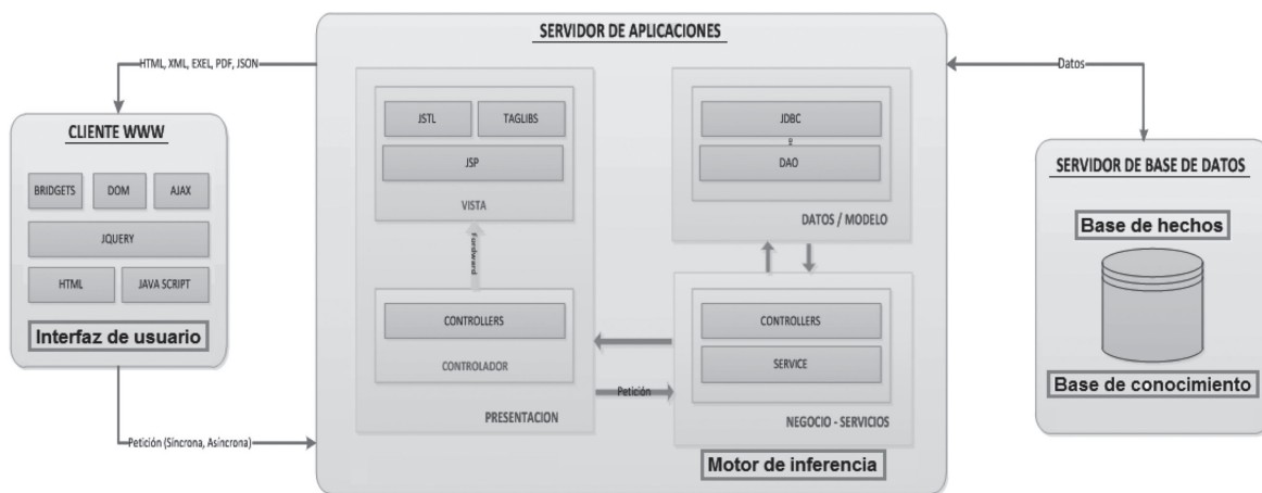
Figura 3. Arquitectura del Sistema.
