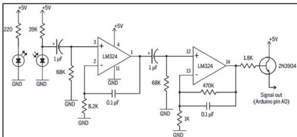
Figura 2. Diagrama de circuito del módulo de ritmo cardiaco.
