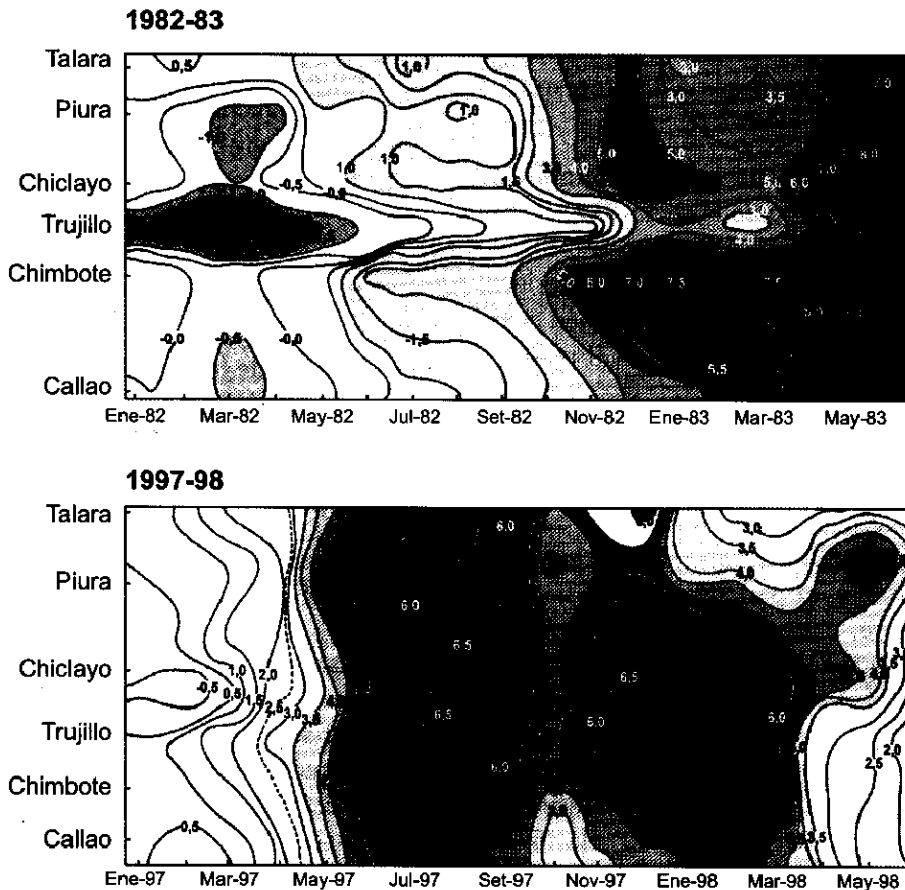
Figura 3. Anomalía de la temperatura mínima (Fuente: http://www.noaa.gov/ ).
