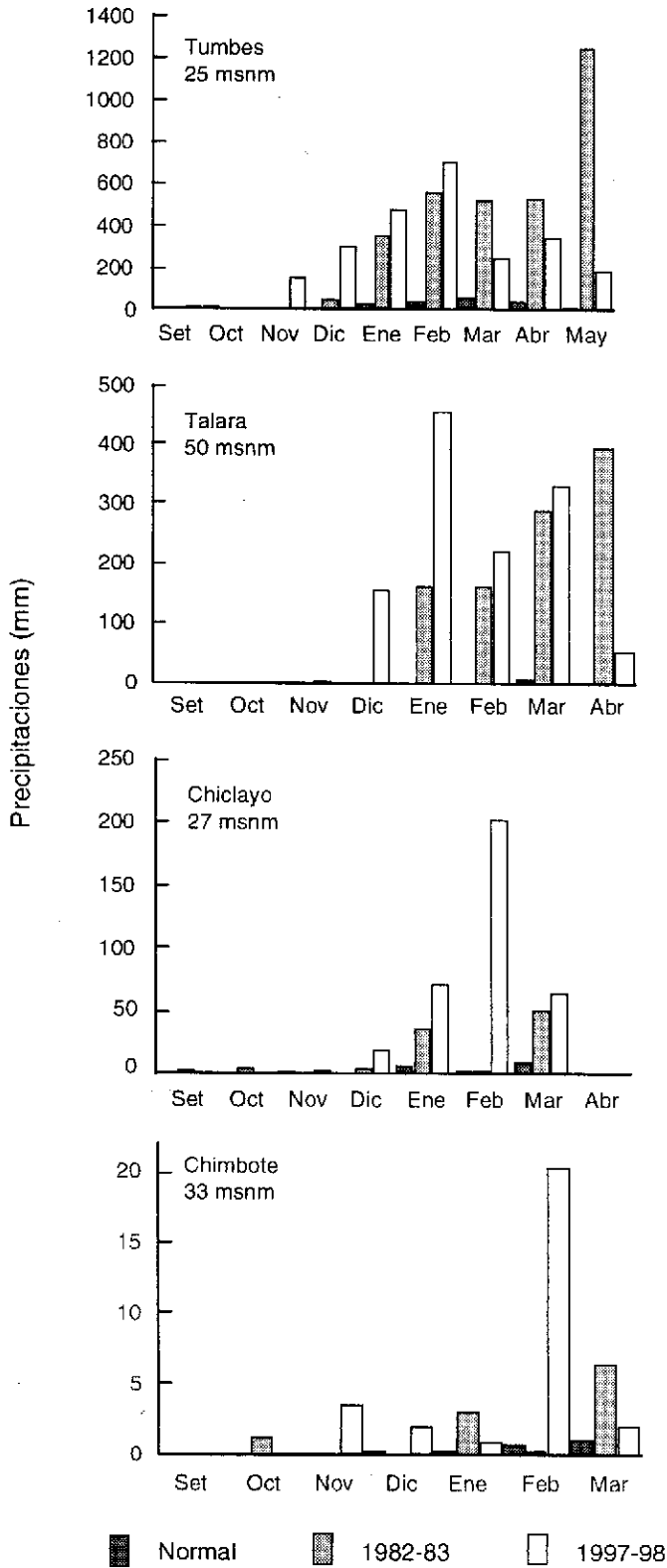
Figura 4. Precipitaciones durante el período lluvioso 1982-83 y 1997-98.
