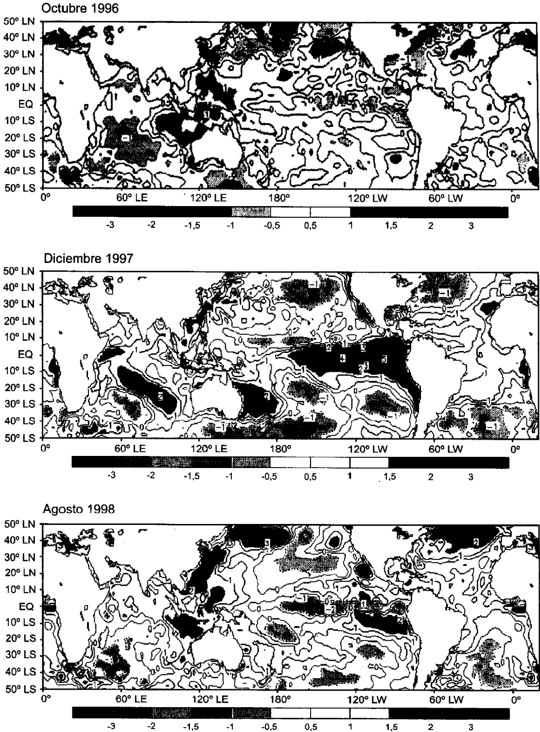
Figura 2. Anomalia de la temperatura superficial del agua de mar (Fuente: http://www.noaa.gov ).
