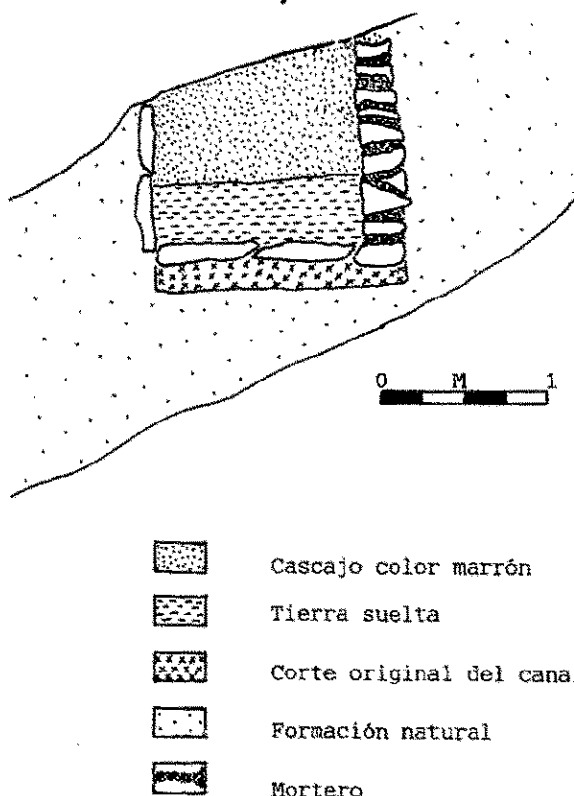
Fig. 3. Diagrama del corte del canal a corta distancia de la laguna de Yanaqocha.
